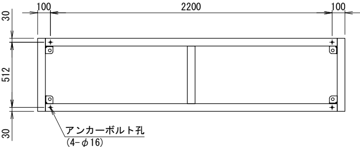
＜アンカー寸法図＞ SCALE= 1:20
