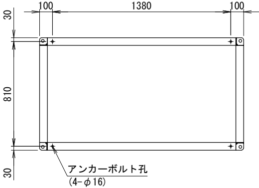
＜アンカー寸法図＞ SCALE= 1:20
