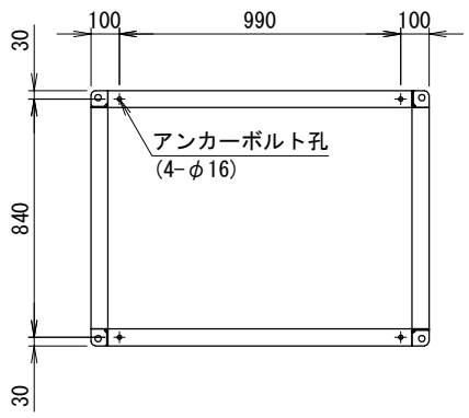
＜アンカー寸法図＞ SCALE= 1:20
