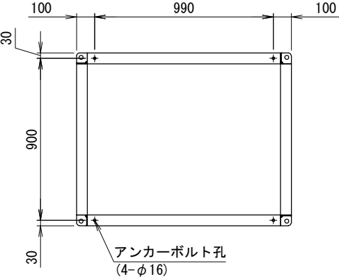
＜アンカー寸法図＞ SCALE= 1:20
