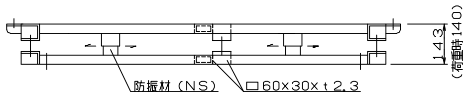
基礎図
