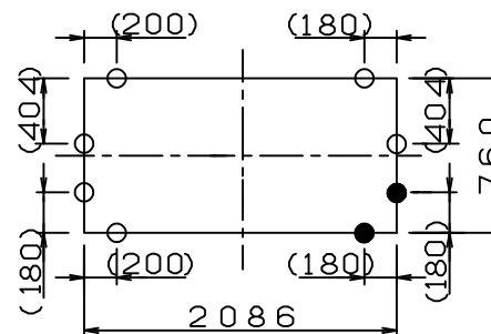
防振材位置
