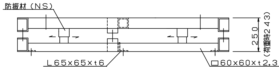
基礎図
