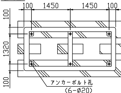
基礎図
