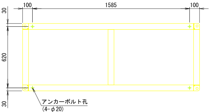
<アンカー寸法図> SCALE= 1:15
