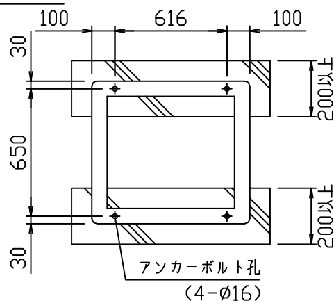
基礎図
