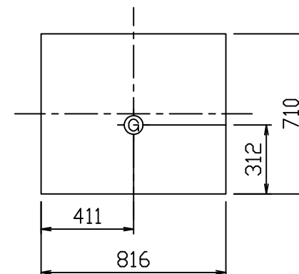
重心位置
