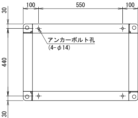
<アンカー寸法図> SCALE= 1:10
