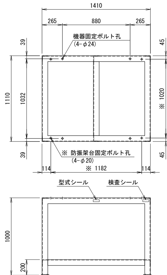
＜アンカー寸法図＞ SCALE= 1:25
