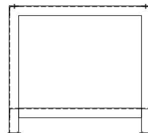
＜アンカー部詳細＞(対面对称形状)
