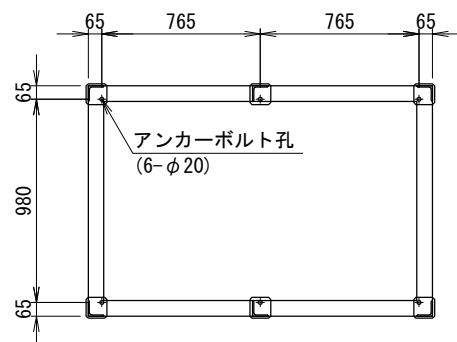
＜アンカー寸法図＞ SCALE= 1:25
