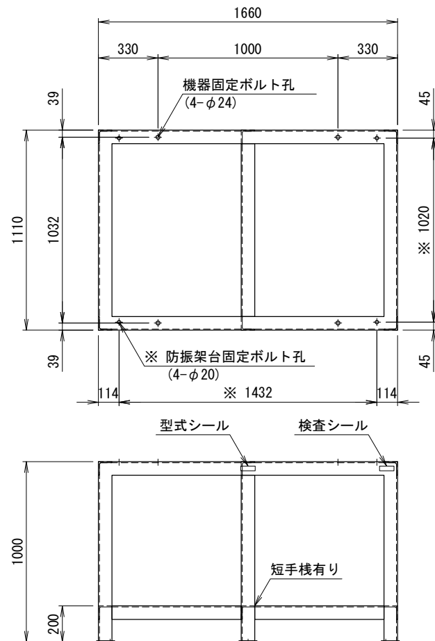
＜アンカー寸法図＞ SCALE= 1:25
