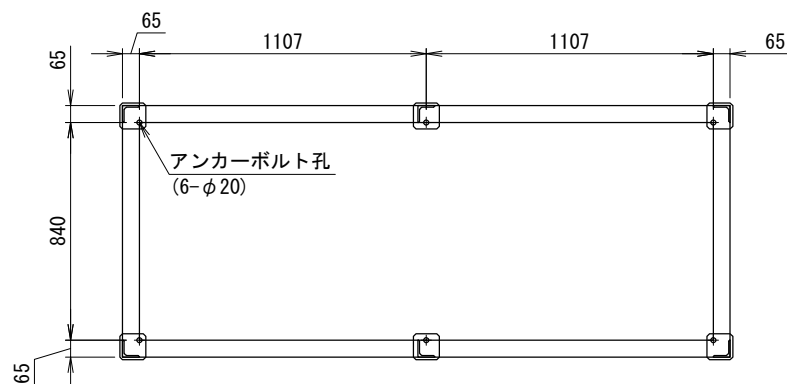
〈アンカー寸法図〉 SCALE= 1:20
