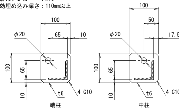
＜アンカ一部詳細＞(対面对称形状)
