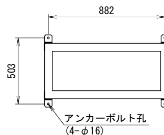
アンカー金具取付 (C)
