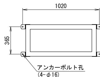
アンカー金具取付 (B)
