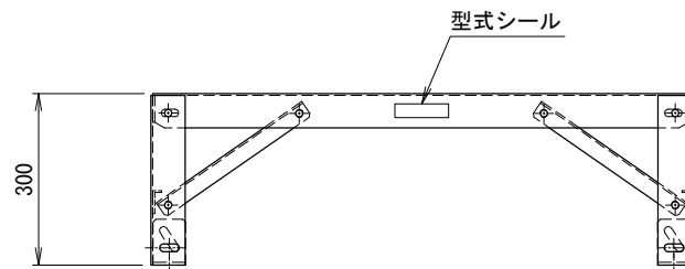
アンカー金具取付 (B)
