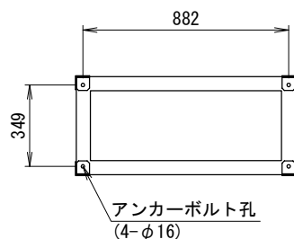
＜アンカー寸法図＞ SCALE= 1:20 アンカー金具取付 (A)
