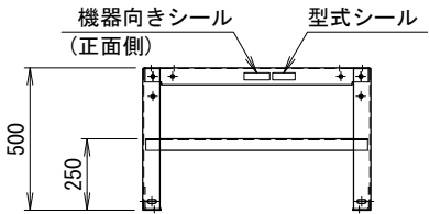
アンカー金具取付 (B)
