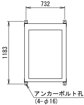
アンカー金具取付 (C)
