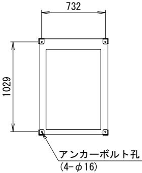
＜アンカー寸法図＞ SCALE = 1:30 アンカー金具取付 (A)
