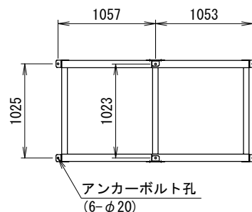
アンカー金具取付 (B)
