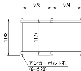
アンカー金具取付 (C)
