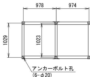
<アンカー寸法図> SCALE = 1:40 アンカー金具取付 (A)
