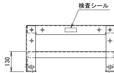
アンカー金具取付 (C)
