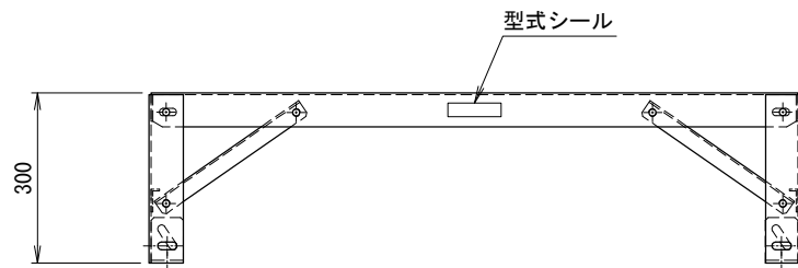
＜アンカー寸法図＞ SCALE= 1:20 アンカー金具取付 (A)
