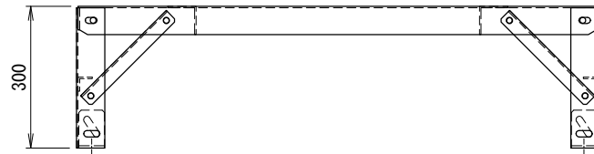
<アンカー寸法図(長孔中心)> SCALE= 1:20 アンカー金具取付(A)内側
