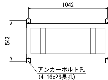
アンカー金具取付(C)外側前後面
