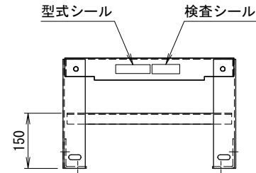
アンカー金具取付(C)外側前後面
