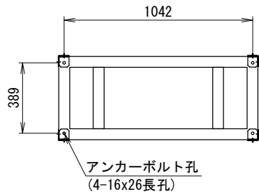
<アンカー寸法図(長孔中心)> SCALE= 1:20 アンカー金具取付(A)内側
