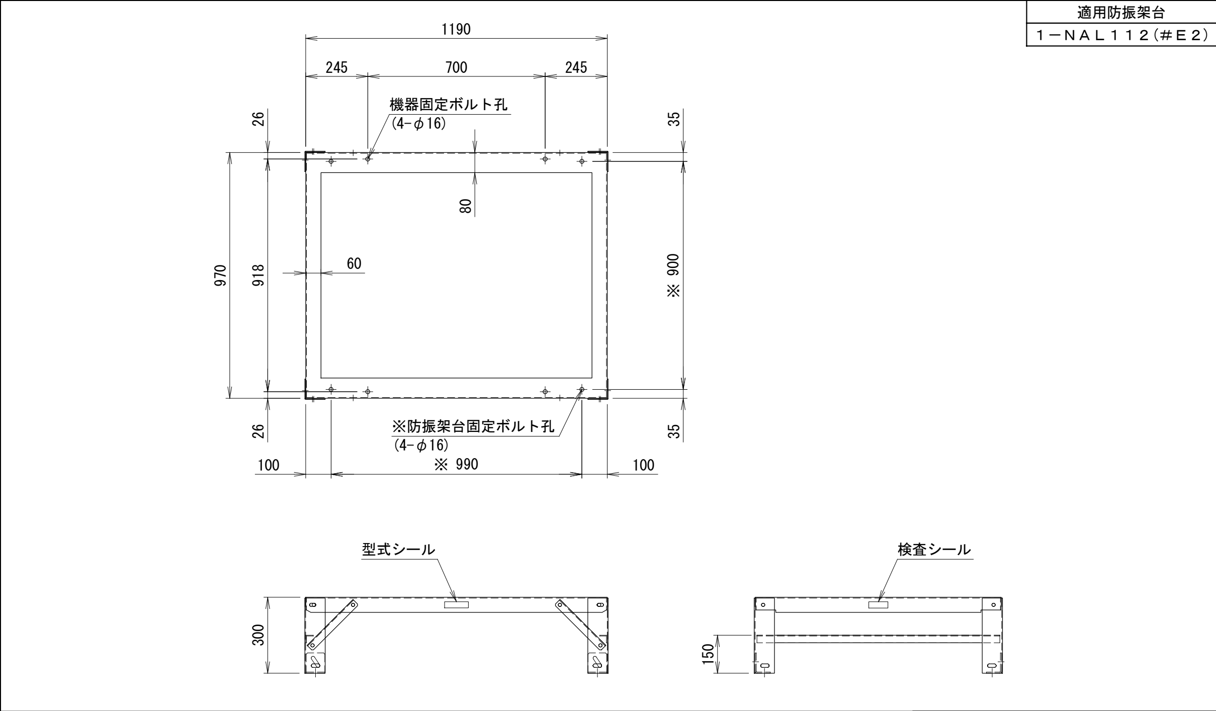
＜アンカー寸法図(長孔中心)＞ SCALE= 1:30 アンカー金具取付(A)内側
