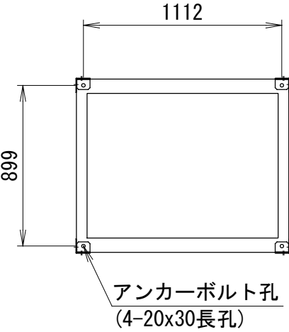
＜アンカー寸法図(長孔中心)＞ SCALE= 1:30 アンカー金具取付(A)内側
