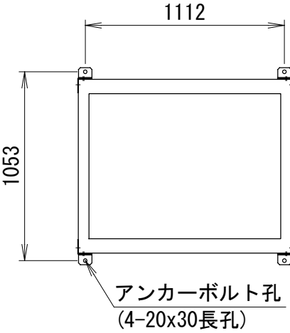
アンカー金具取付(C)外側前後面
