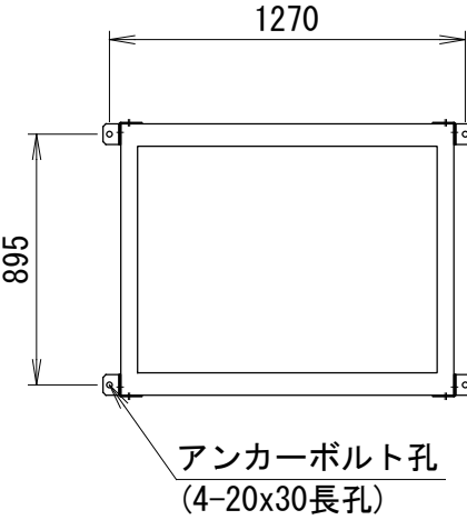
アンカー金具取付(B)外側側面
