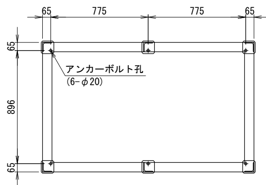
<アンカー寸法図> SCALE= 1:20
