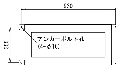
アンカー金具取付 (B)
