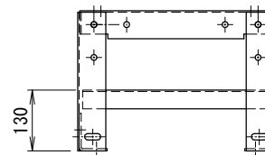
アンカー金具取付 (C)
