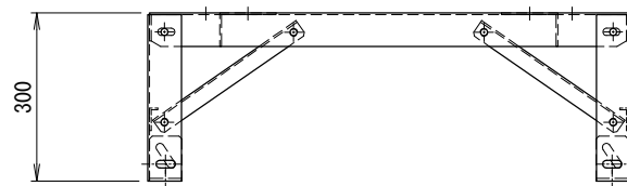
アンカー金具取付 (B)
