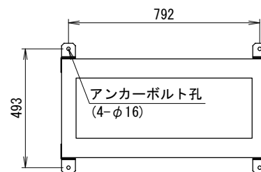
アンカー金具取付 (C)
