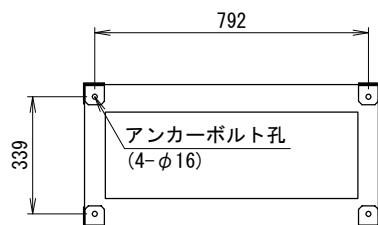
＜アンカー寸法図＞ SCALE= 1:15 アンカー金具取付 (A)
