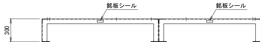
〈アンカー寸法図〉 SCALE= 1:20
