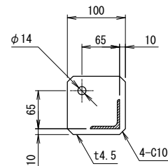
＜アンカー部詳細＞(対面对称形状) アンカーボルト参考 接着系アンカー : M10 有効埋め込み深さ : 80mm以上
