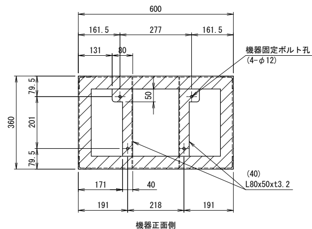
機器正面側
