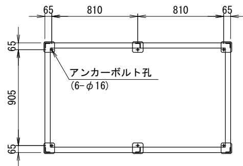
＜アンカー寸法図＞ SCALE= 1:25
