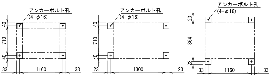
アンカー金具取付 (A)
