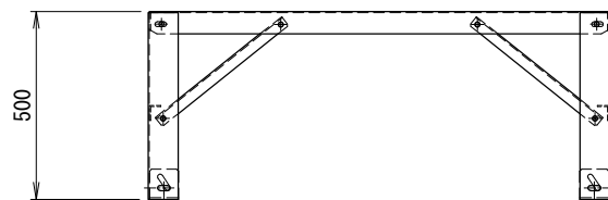
アンカー金具取付 (B)
