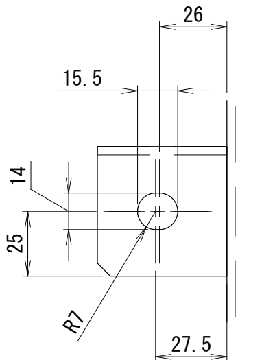
機器固定ボルト孔 (A部) 詳細図 (SCALE=1:2)
