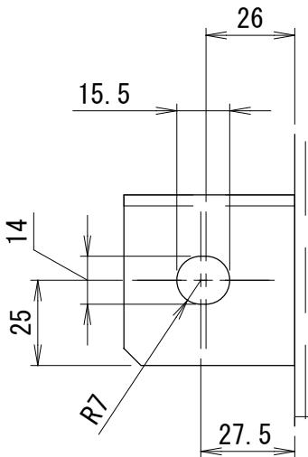
機器固定ボルト孔(A部)詳細図 (SCALE=1:2)
