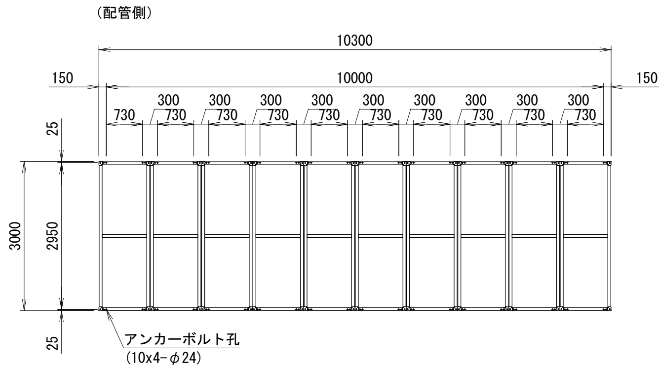
＜アンカー寸法図（下ベース基準）※A孔＞
