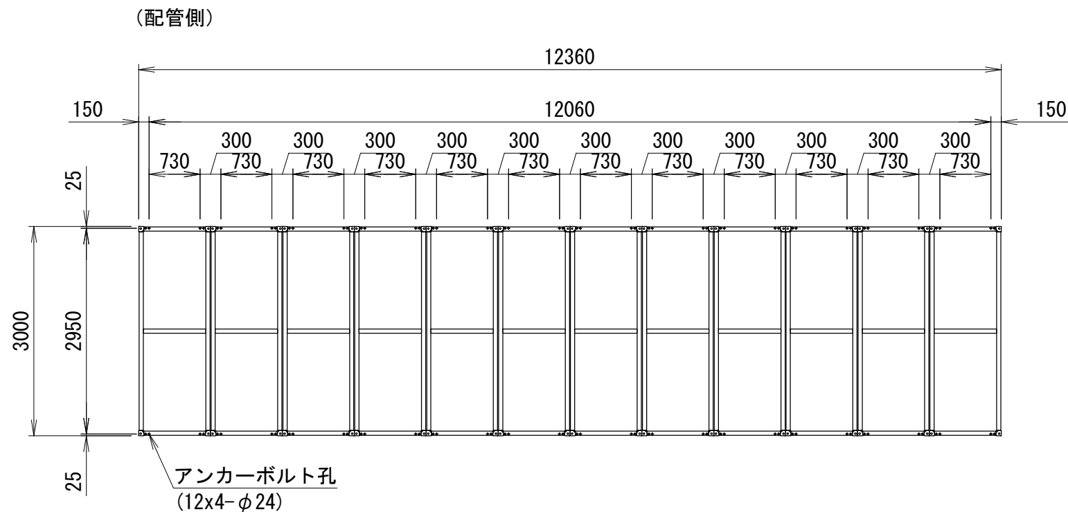
＜アンカー寸法図（下ベース基準）※A孔＞
