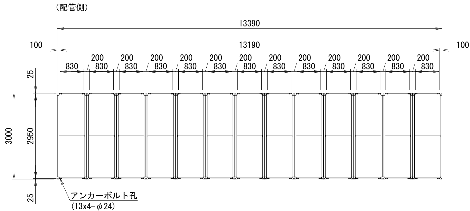
＜アンカー寸法図（下ベース基準）※B孔＞
