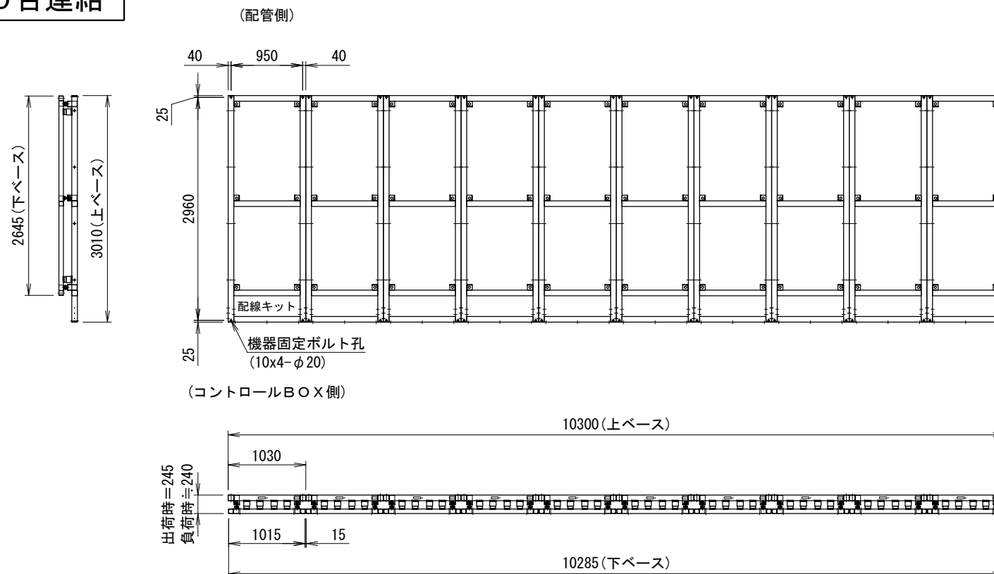
＜アンカー寸法図（下ベース基準）＞
