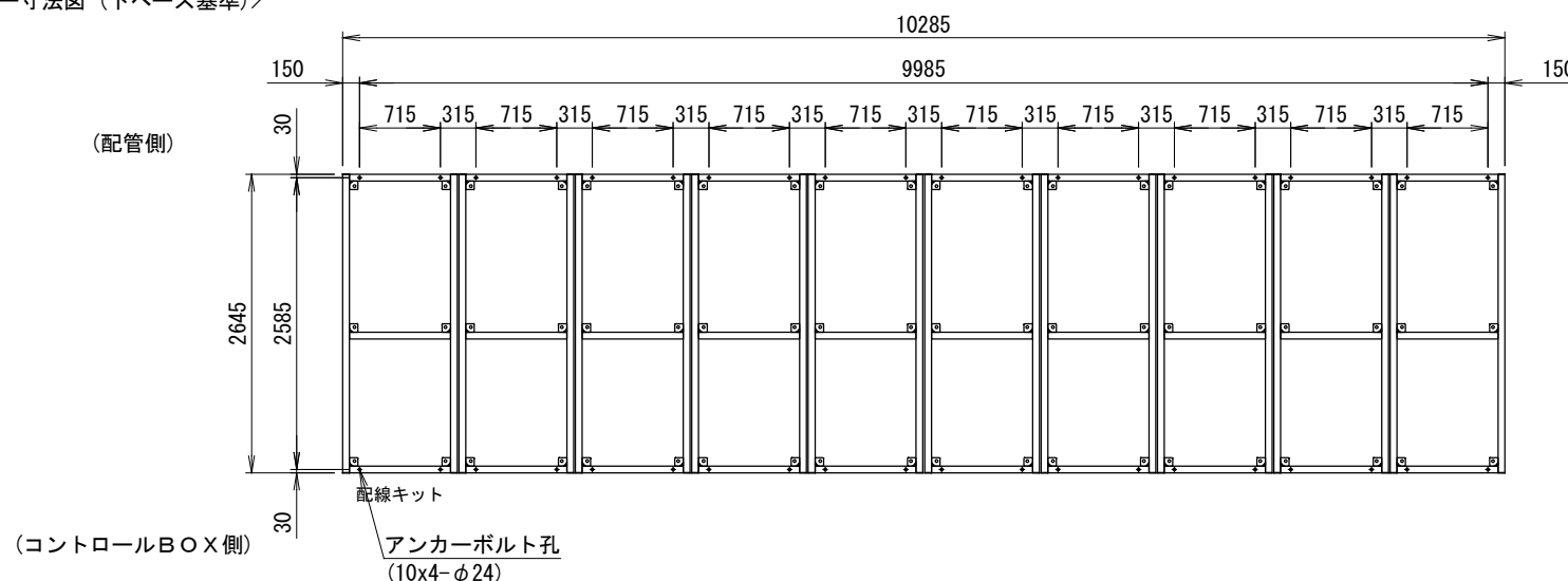
＜アンカー寸法図（下ベース基準）＞
