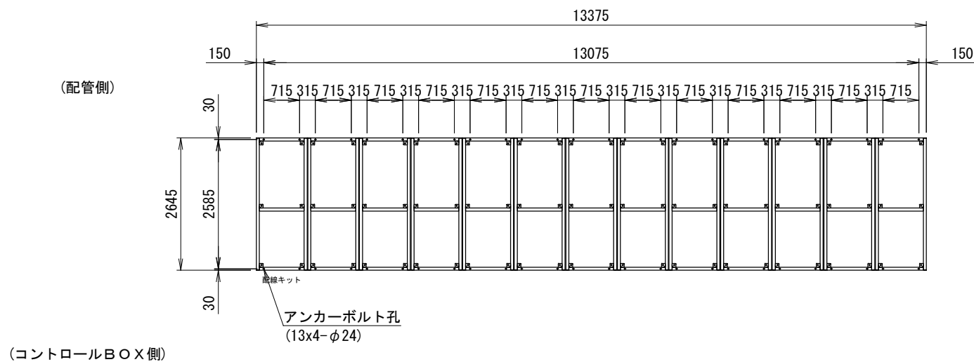
〈アンカー寸法図（下ベース基準）〉
