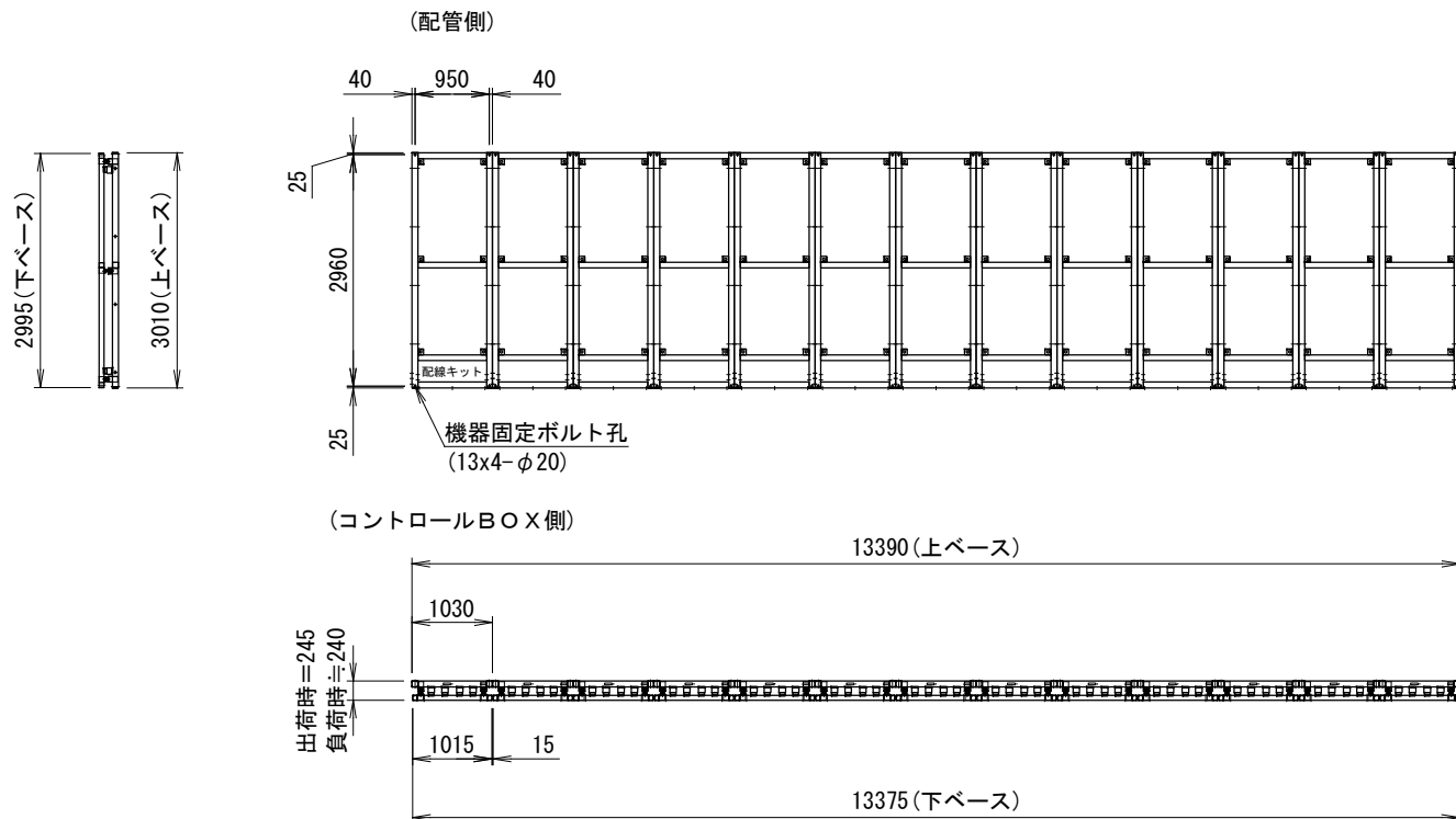
〈アンカー寸法図（下ベース基準）〉
