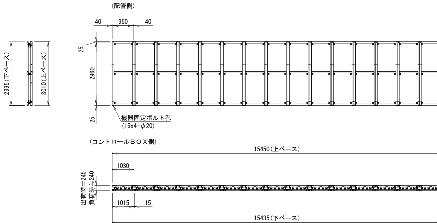
〈アンカー寸法図（下ベース基準）〉
