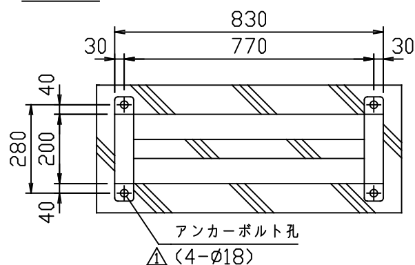
基礎図
